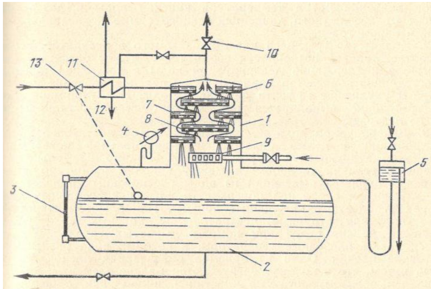
Рисунок 27 – Схема атмосферного деаэратора смешивающего действия
