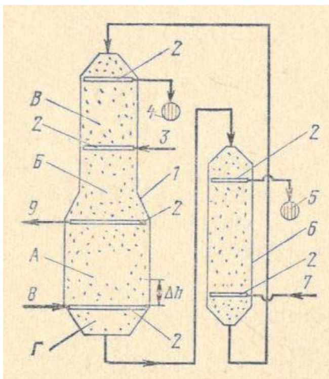
Рисунок 14 – Ионитный фильтр непрерывного действия
